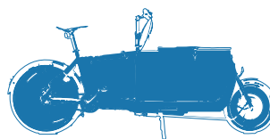
„iBullit“ Beispiel für ein Lastenrad-Pedelec Geschwindigkeit: max. 32 km/h, in Deutschland 25 km/h
