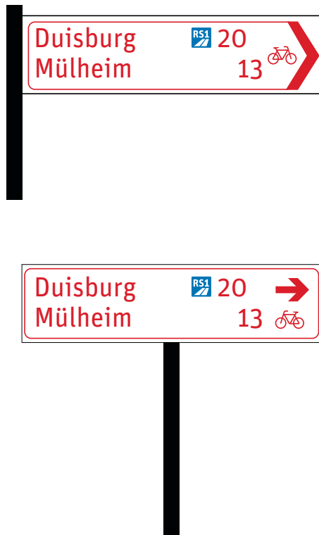
Beispielhafte Anwendung der wegweisenden Beschilderung des Landes NRW (HBR NRW) für den Radschnellweg
