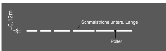
Schutzmarkierung zur Verdeutlichung von Pollern
